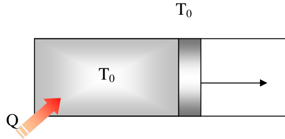
شکل ۵-۳۲. فرآیند برگشت پذیر انبساط همدمما
